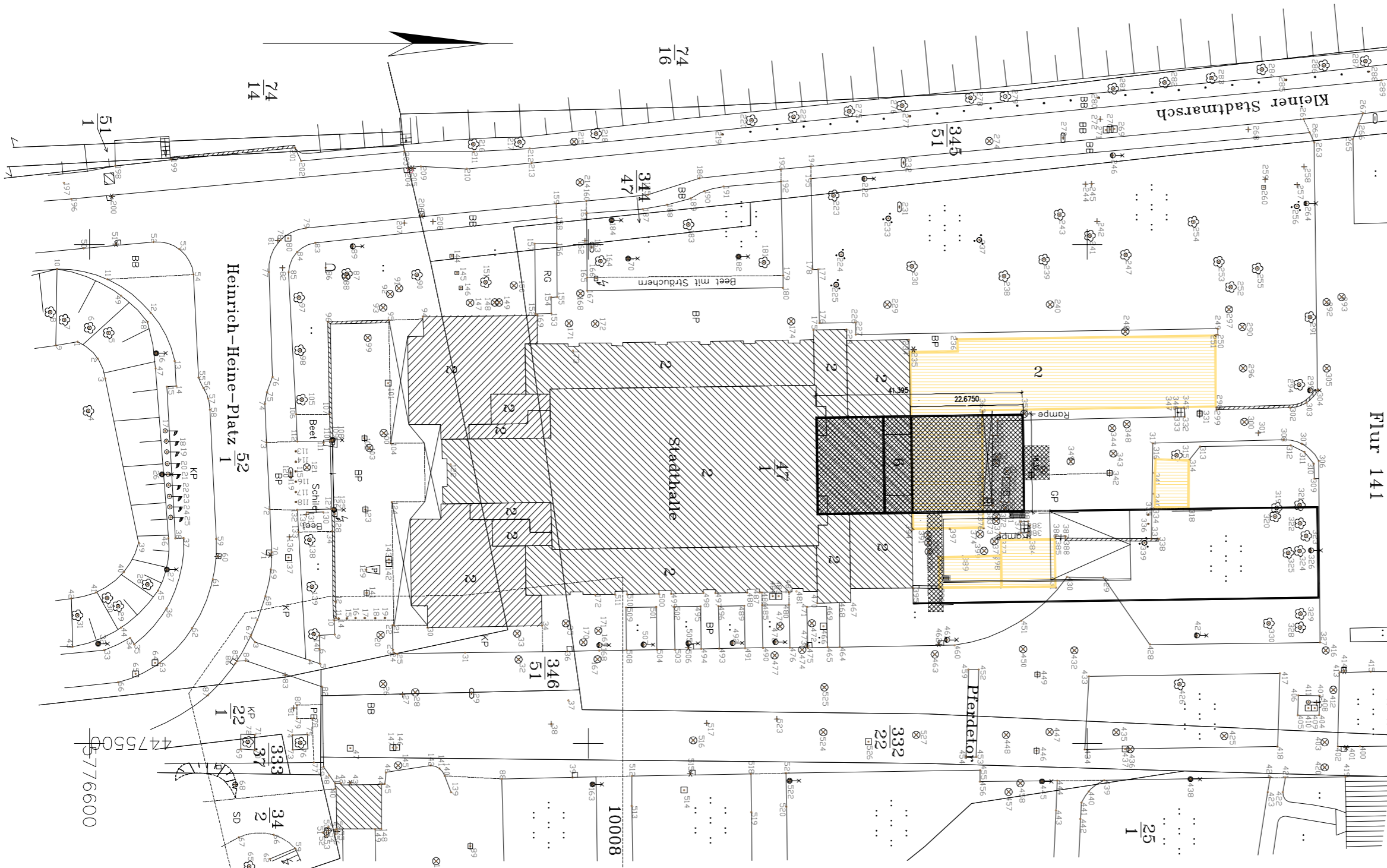
Gebäudebesicht AC1-100.00
