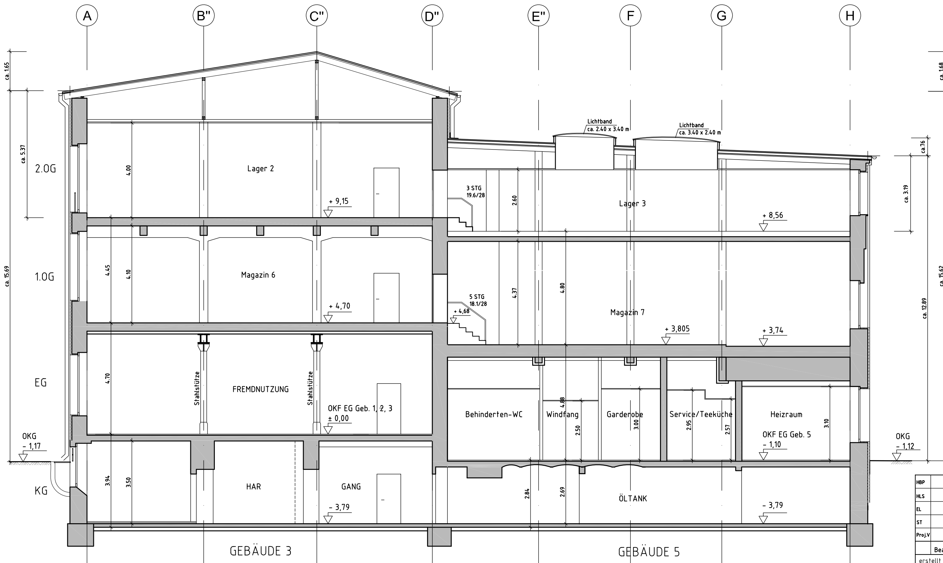
SCHNITT C-C
