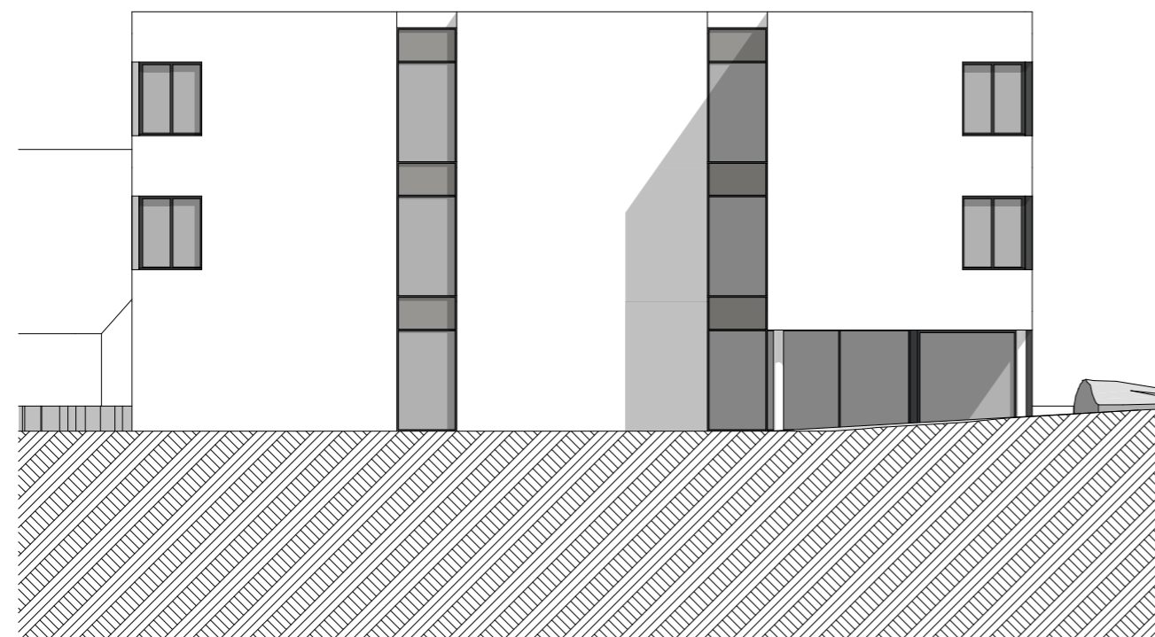
Ansicht Ost
