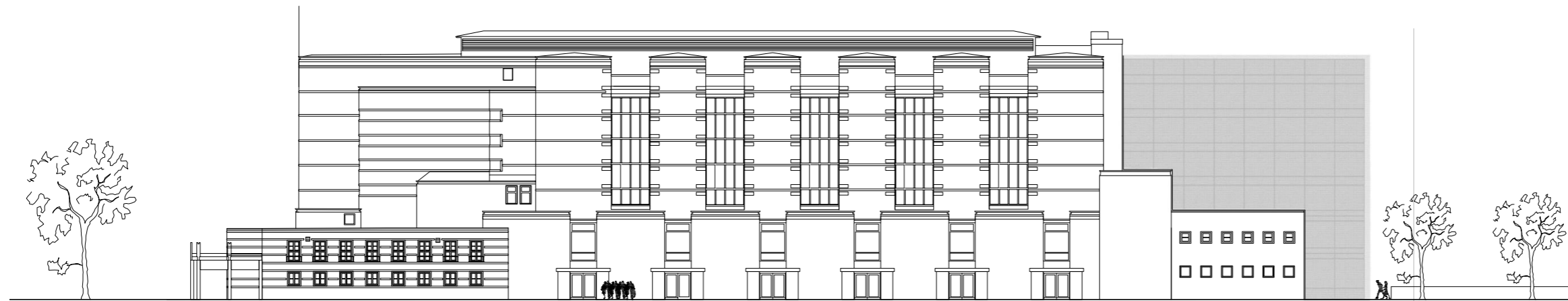
Gebäudeoberseite
