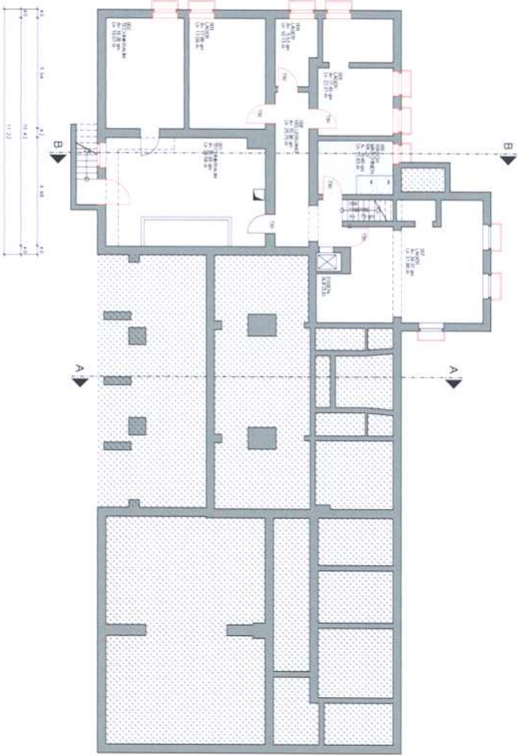
GRUNDRISS KELLERGEESCHOSS
