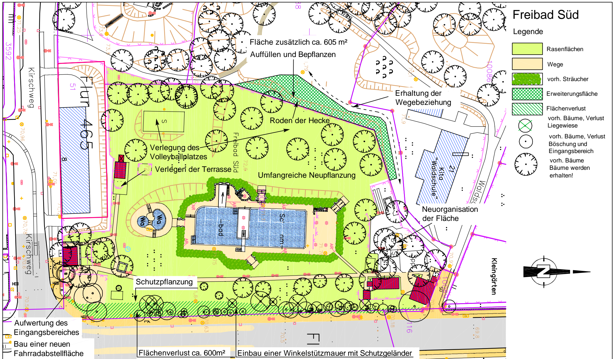
DS0590/08 Anlage 6 Bestands- und Maßnahmenplanung für Variante 1 M 1 : 1000
