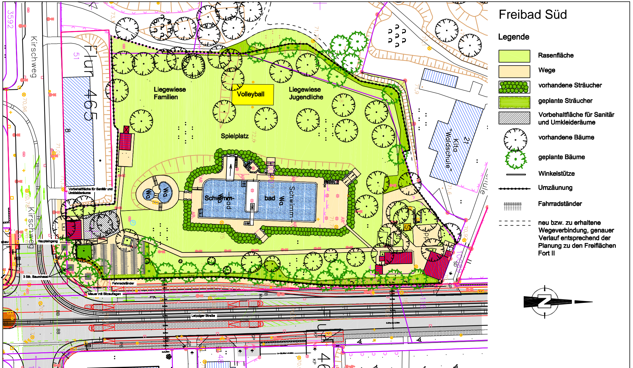
DS0590/08 Anlage 7 Entwicklungsplan für Variante 1 M 1 : 1000
