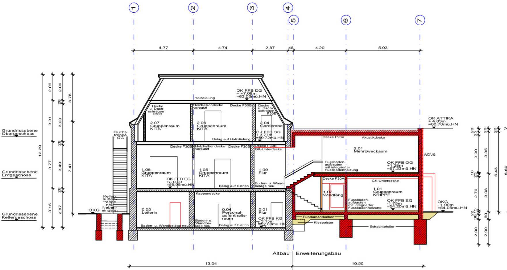
KITA "Bertis Biberburg" - Schnitt A - A
