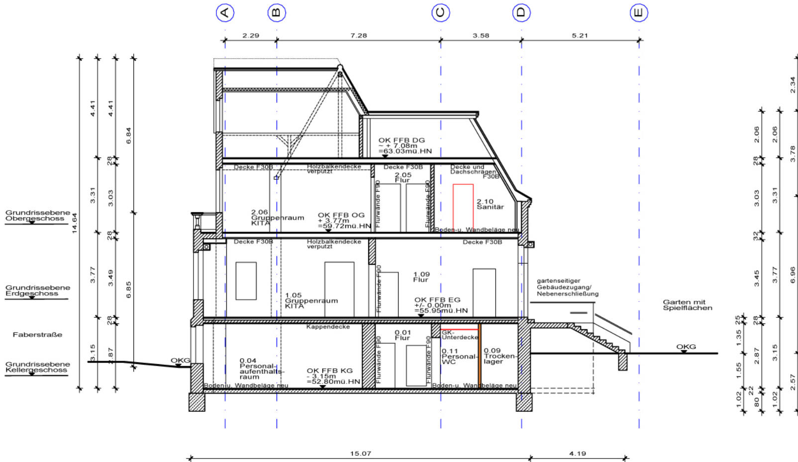
KITA " Bertis Biberburg " - Schnitt B - B
