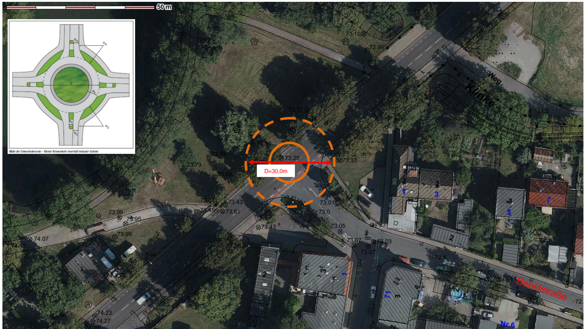
Skizzenhafte Einordnung eines kleinen Kreisverkehrs (Außendurchmesser 30,0m) ohne die Einordnung von Nebenanlagen, wie z.B. Gehwege und Radwege
